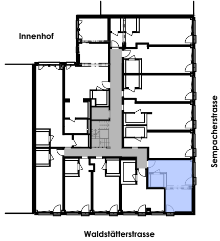
Grundriss
